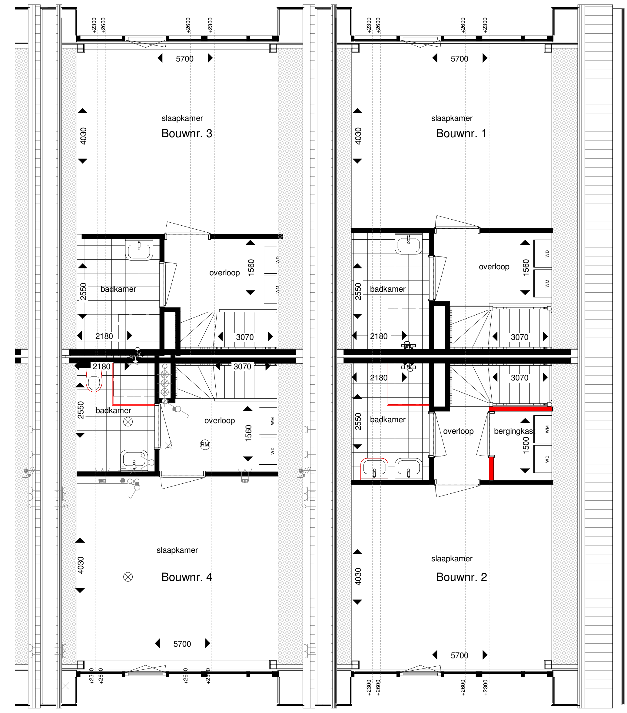
1e Verdieping SCHAAL 1 : 50
