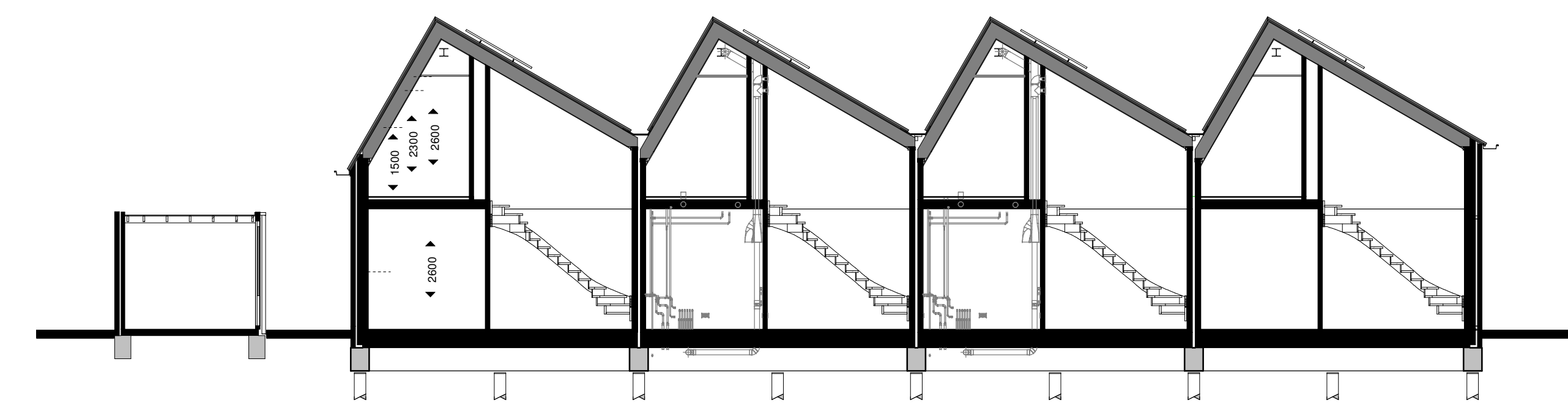
Doorsnede SCHAAL 1 : 100
